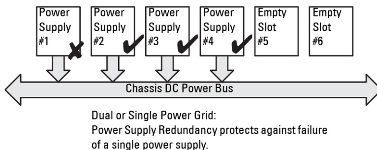
図 15. 電源装置の冗長性 : 合計 4 台の PSU があり、そのうち 1 台が故障。
